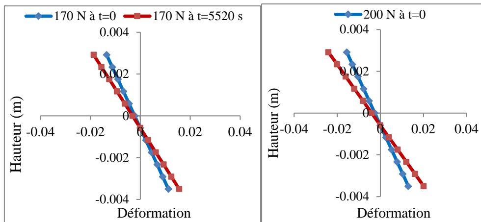
Fig. 7. Répartition des déformations dans la section la plus sollicitée.
