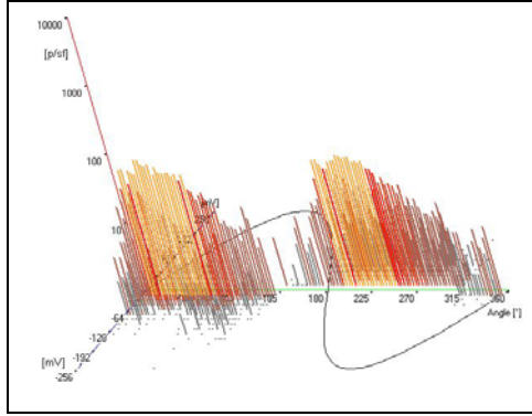
Fig. 7. HG 4 CHE Vidraru 3D – 2009
