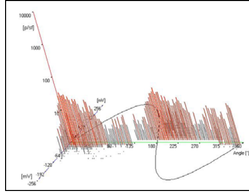
Fig. 8. HG 4 CHE Vidraru 3D - 2010
