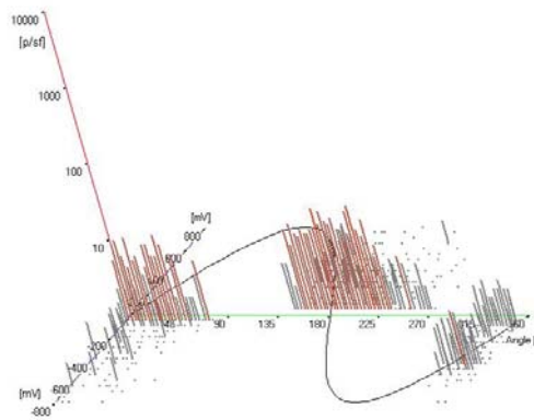
Fig. 10. HG 2 CHE Remeti 3D - 2010
