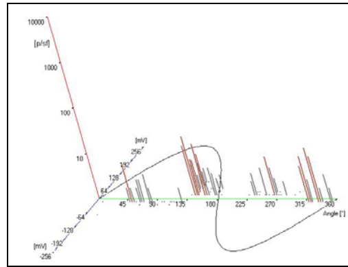
Fig. 13. HG2 CHE Munteni 3D - 2010
