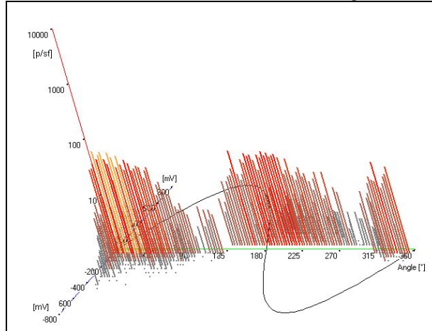
Fig. 5. HG2 CHE Mărișelu 3D - 2010
