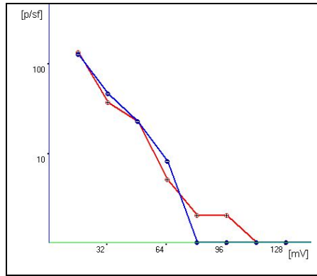
Fig. 11. HG2 CHE Munteni 2D - 2010
